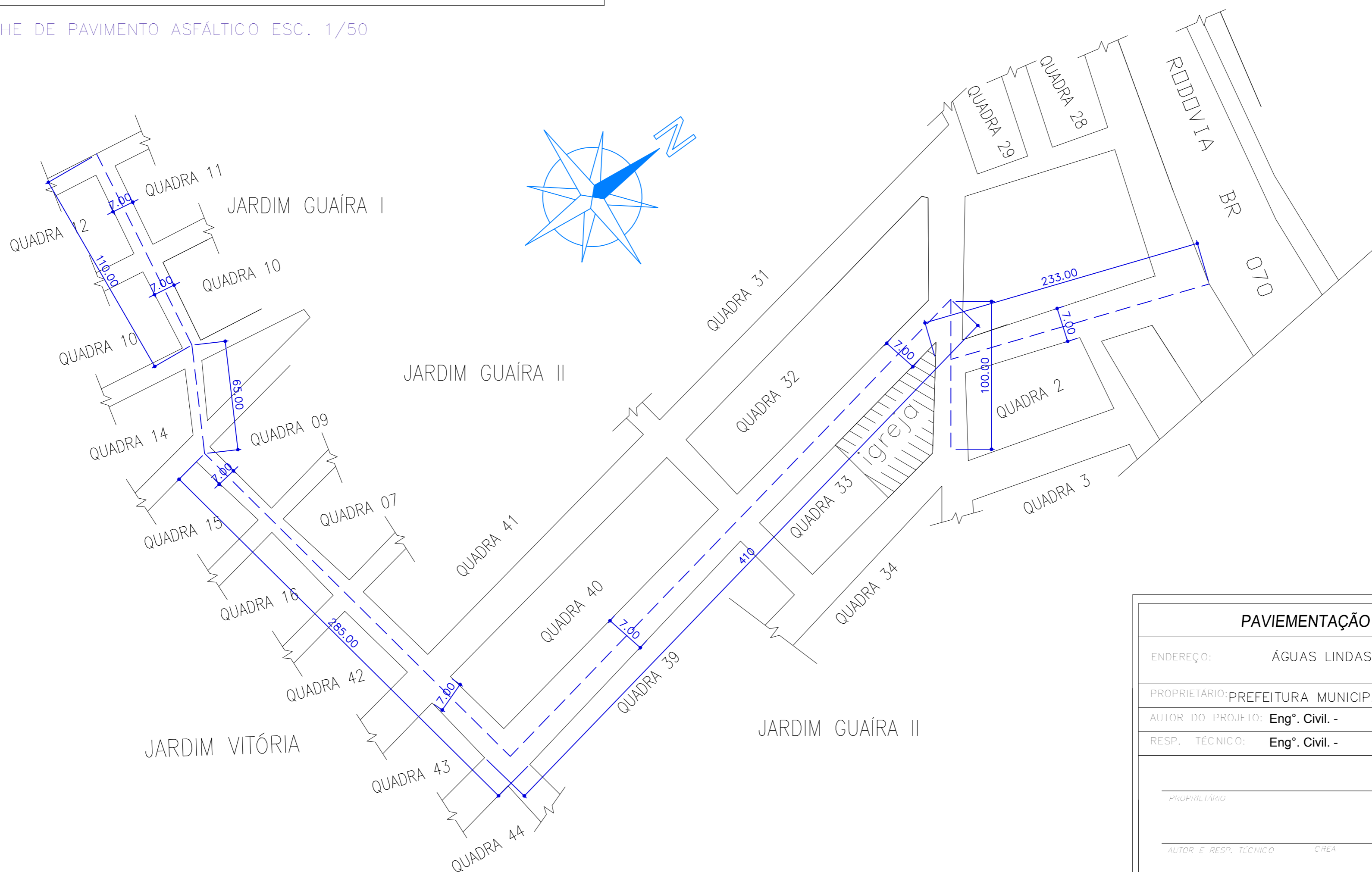
PAVIMENTAÇÃO ASFÁLTICA TRECHO 04 SEM ESCALA
