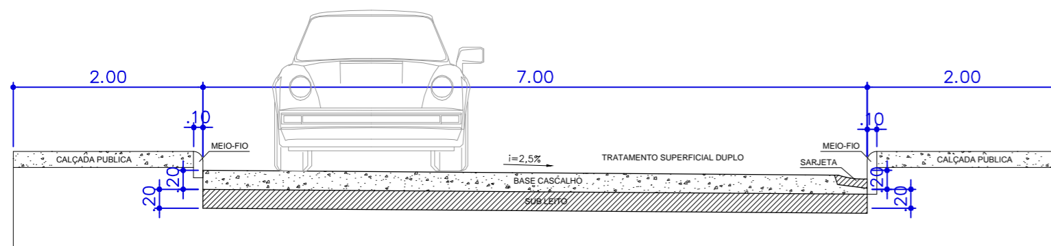
DETALHE DE PAVIMENTO ASFÁLTICO ESC. 1/50
