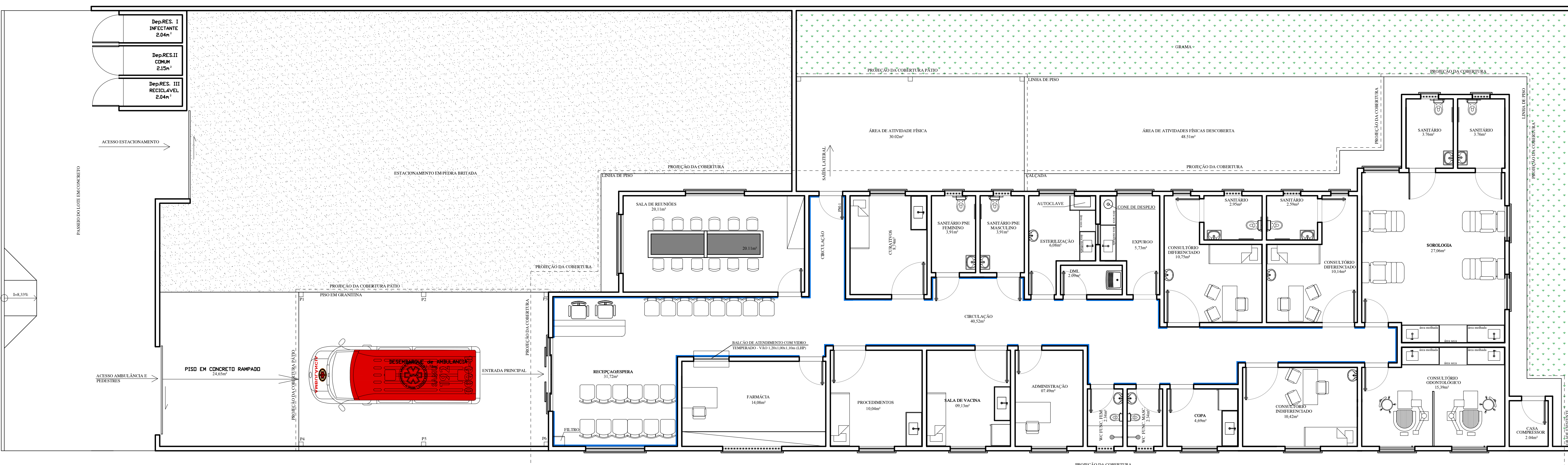
PLANTA DE LAYOUT ESC: 1/75
