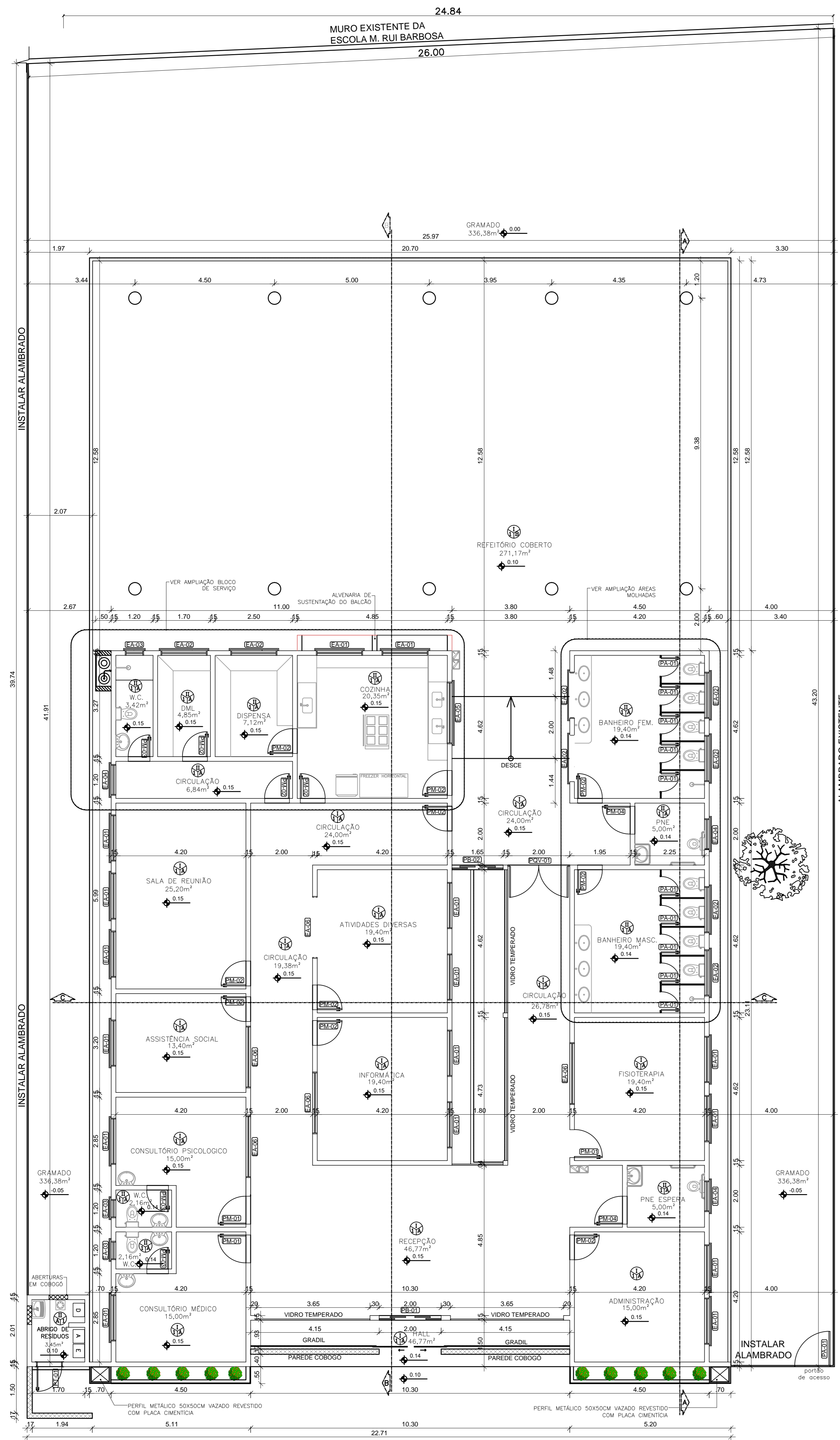
PLANTA BAIXA ESC. 1/75
