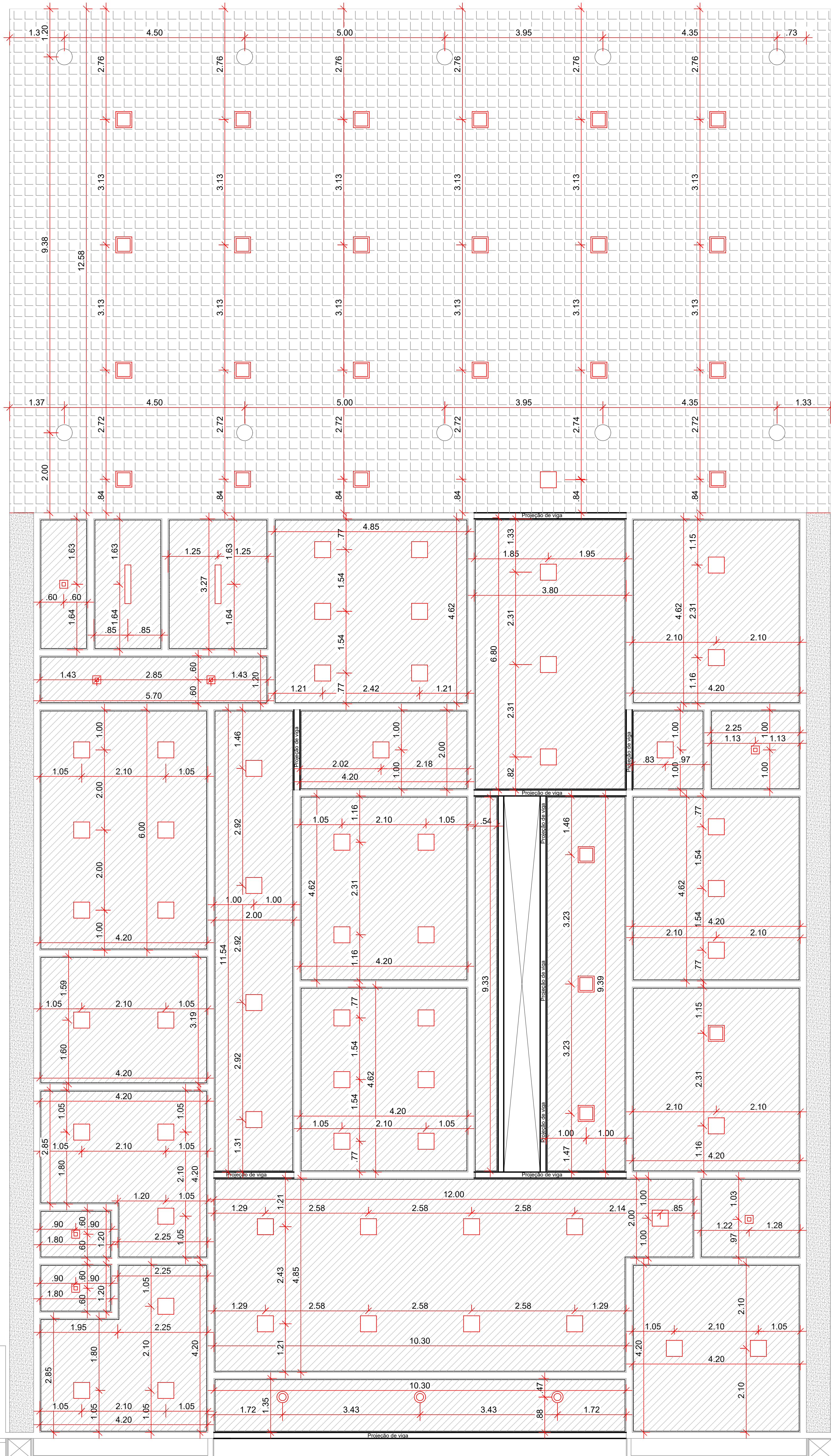
PLANTA DE FORRO ESC. 1/50
