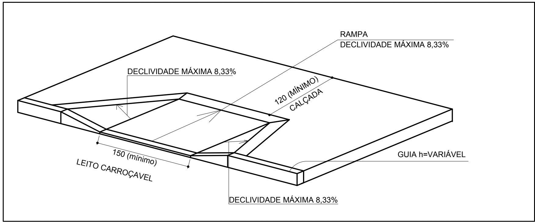
DET. 01 - RAMP A DE ACESSIBILIDADE - CALÇADAS SEM ESC.
