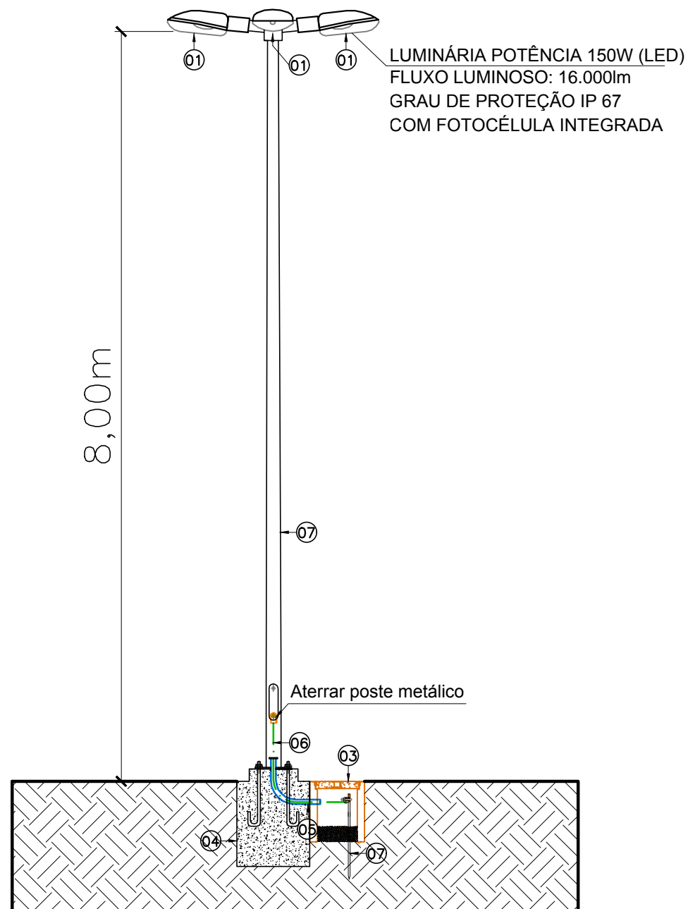
DETALHE DE INSTALAÇÃO DO POSTE SEM ESCALA
