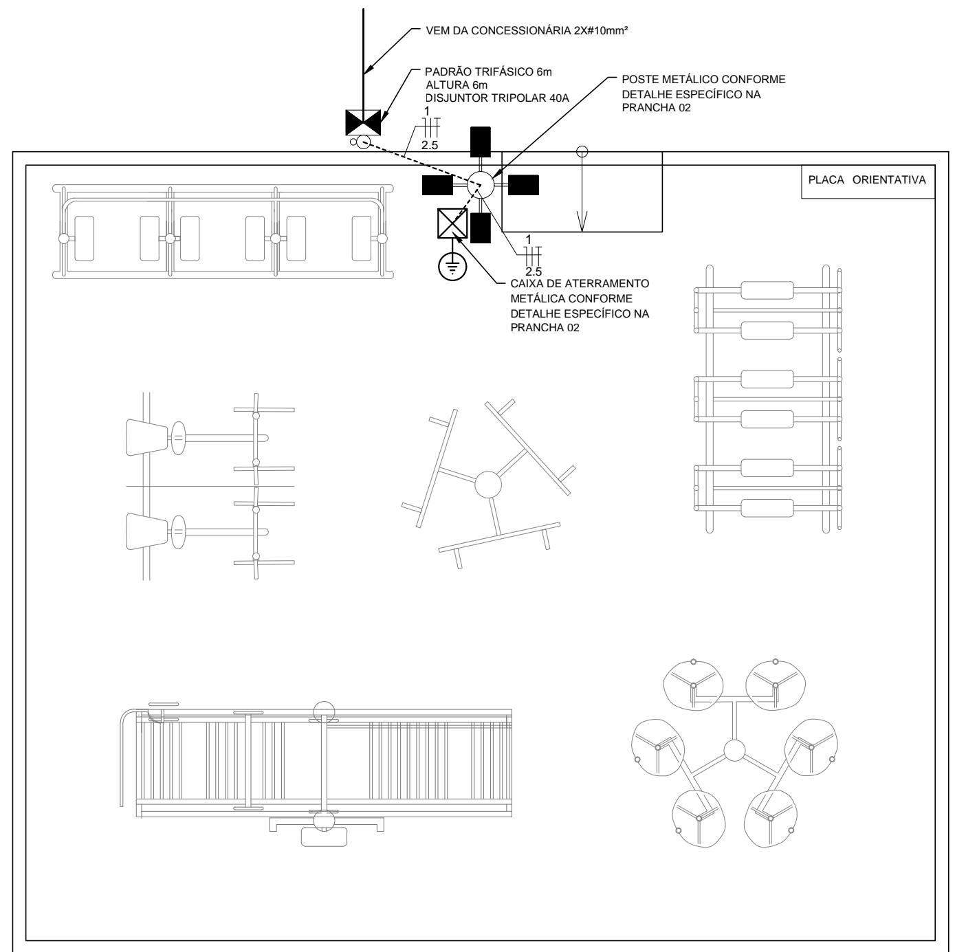
PLANTA BAIXA - LOCAÇÃO DO POSTE SEM ESCALA
