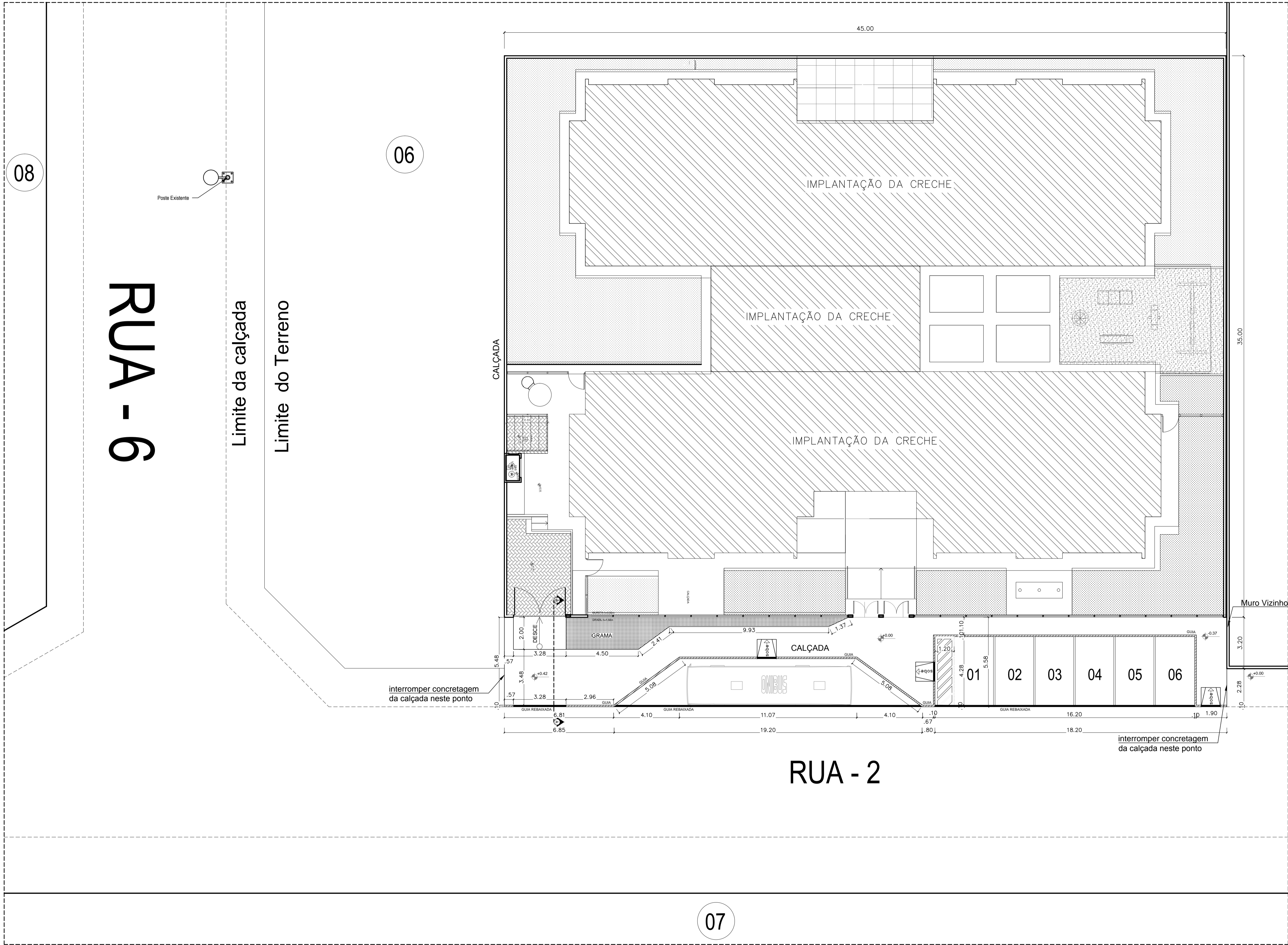
PLANTA BAIXA DE IMPLANTAÇÃO Esc. 1/100
