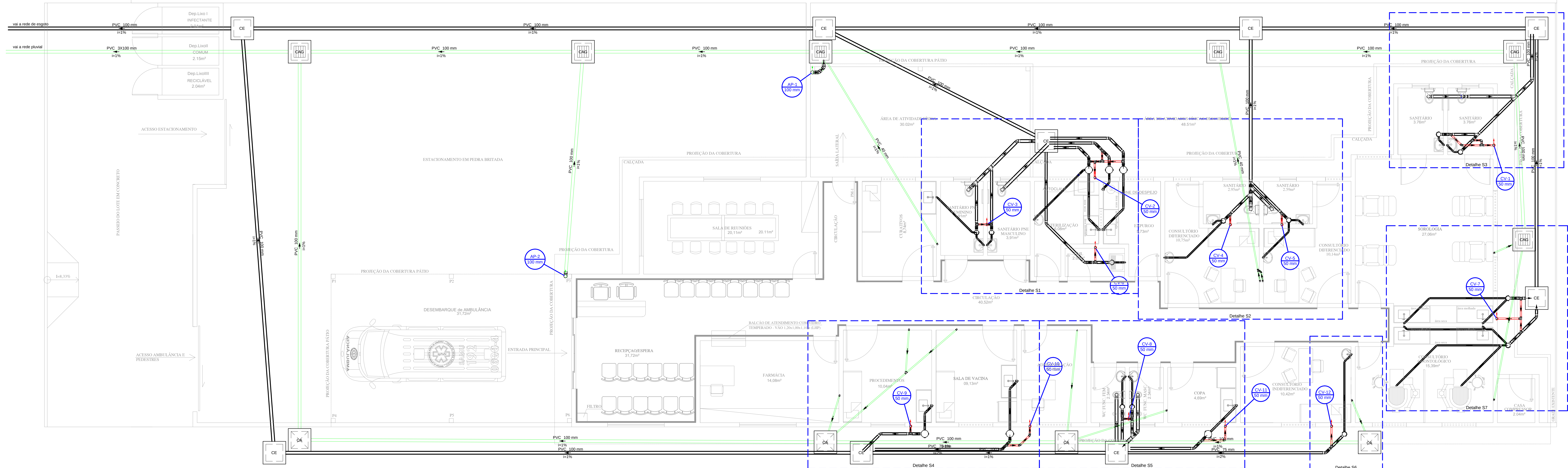
PLANTA SANITÁRIO - TÉRREO escala 1:50
